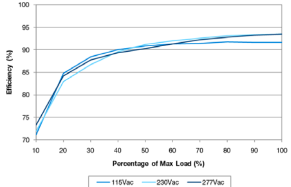
LNE-48V150W□
